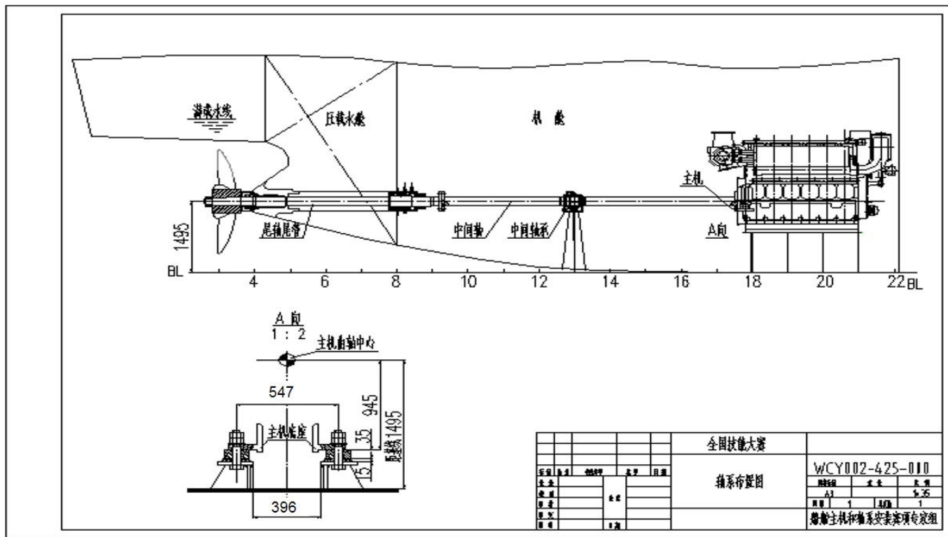
图 1 轴系布置图
